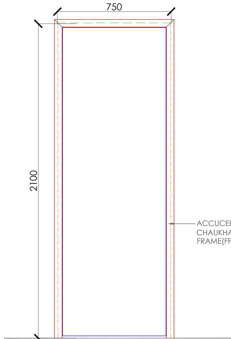
FRAME ELEVATION
